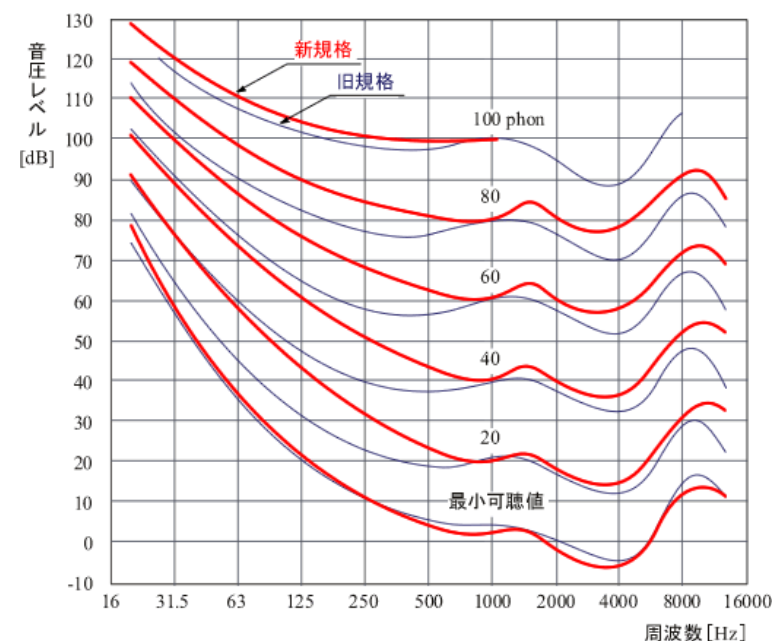
等感曲線
